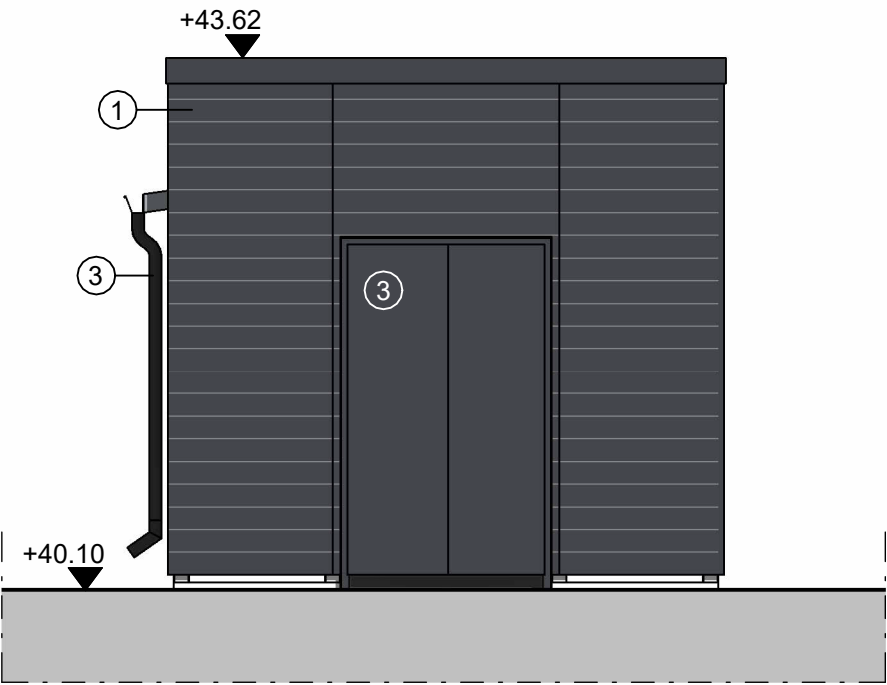
Jätekatos julkisivu luoteeseen 1 : 50
