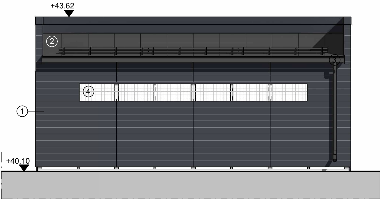
Jätekatos, julkisivu koilliseen 1 : 50
