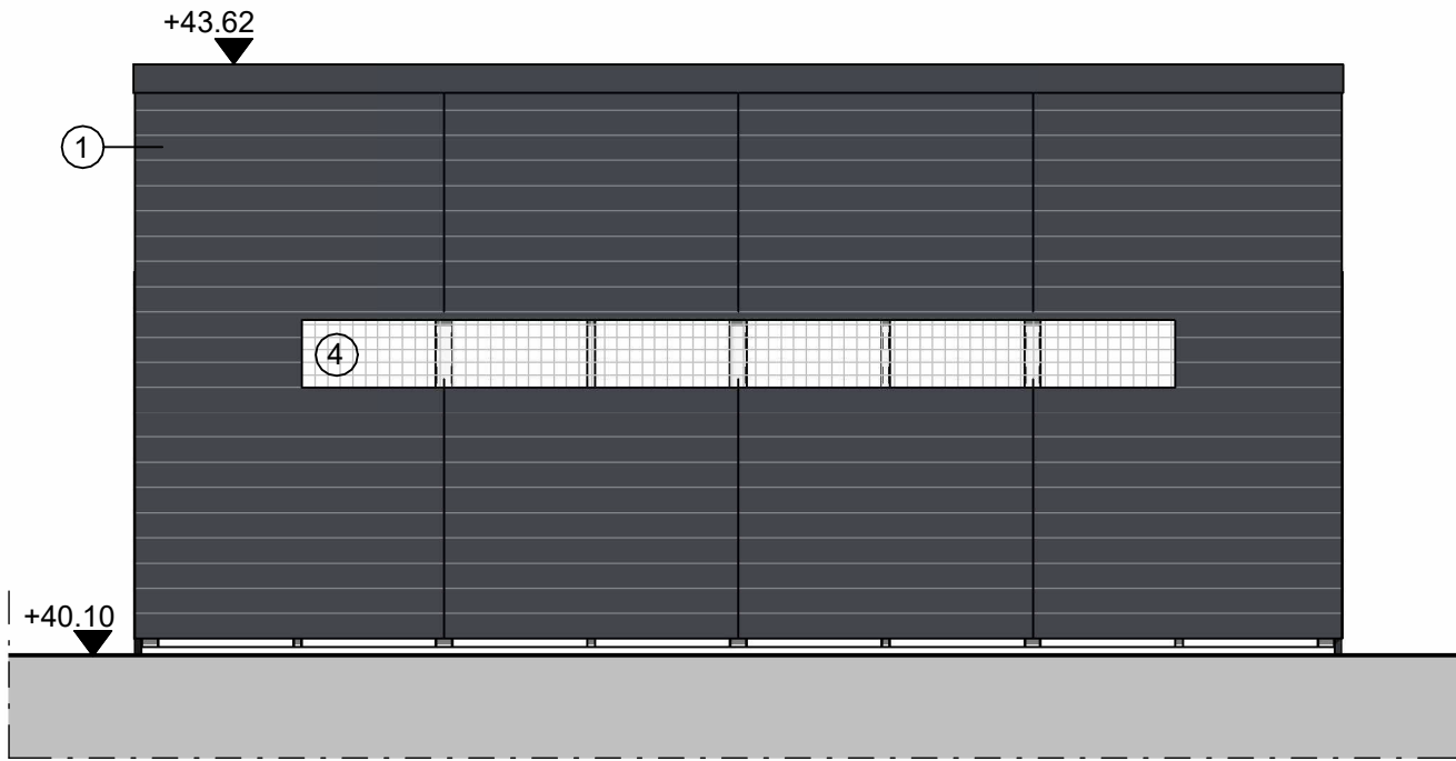
Jätekatos julkisivu lounaaseen 1 : 50
