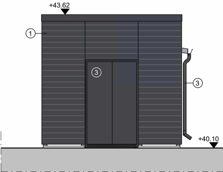
Jätekatos julkisivu kaakkoon 1 : 50
